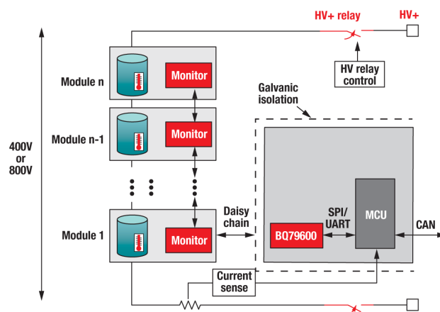
图 1. 分布式 BMS 示例。
