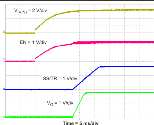
图 8-6. Power Up V_O , V_{(IN)}
