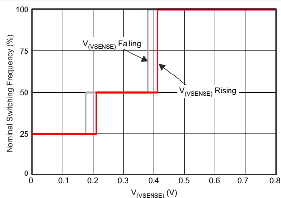
图 6-6. Switching Frequency vs V_{VSENSE}
