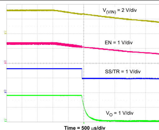
图 8-7. Power Down V_O , V_{(IN)}
