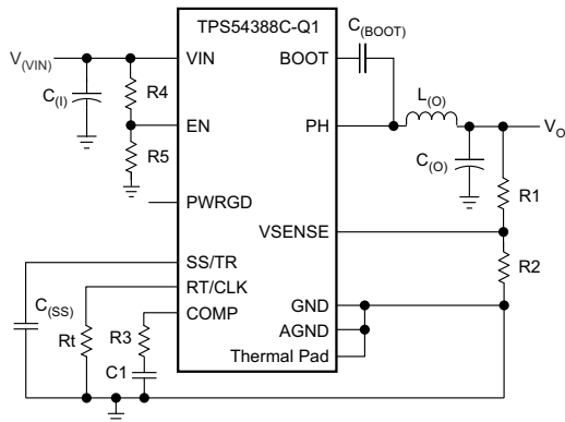
简化原理图
