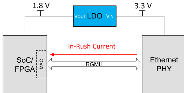
图 8-4. PHY 上电后流入 MAC I/O 引脚的残余电流
