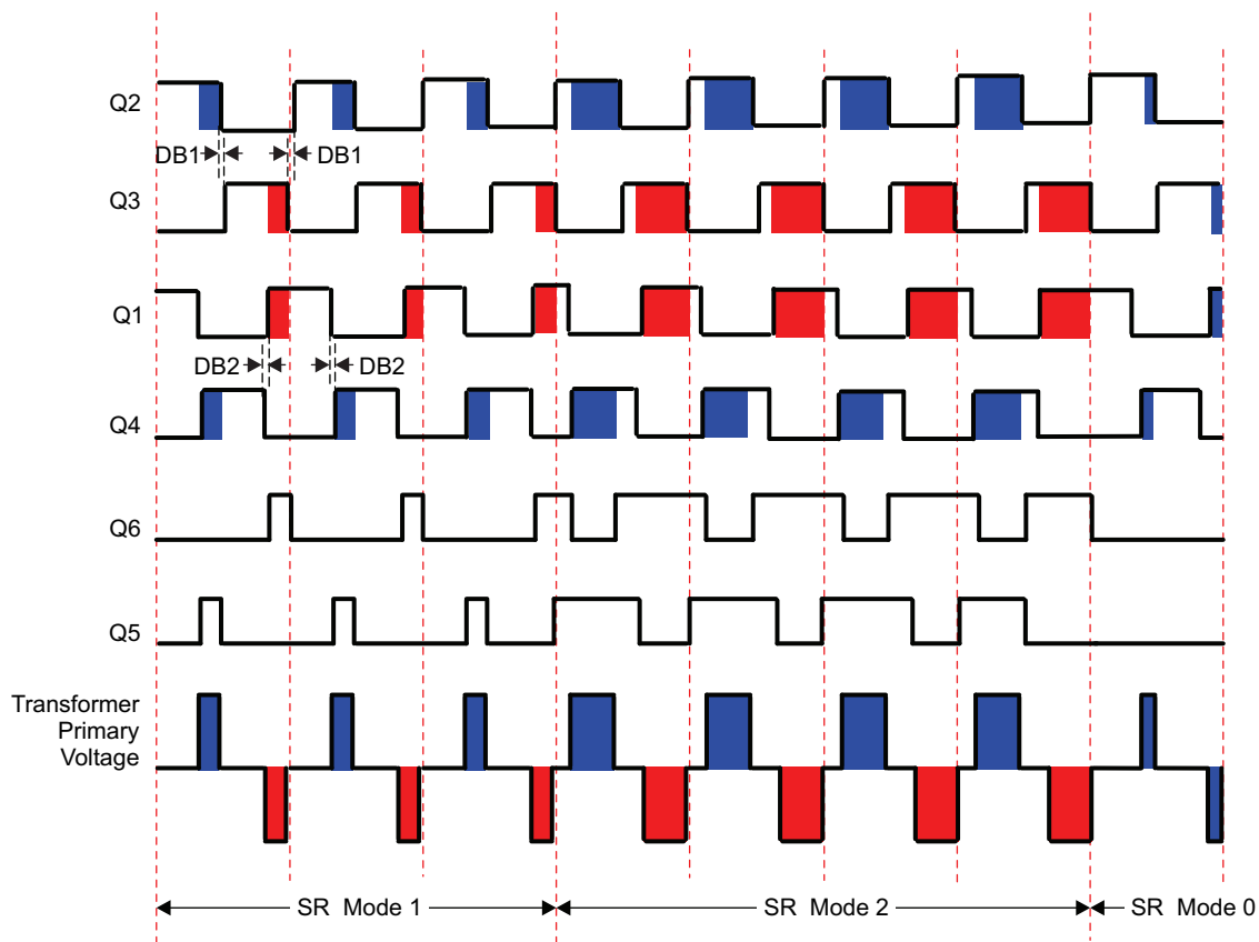
图 14. VMC 波形
