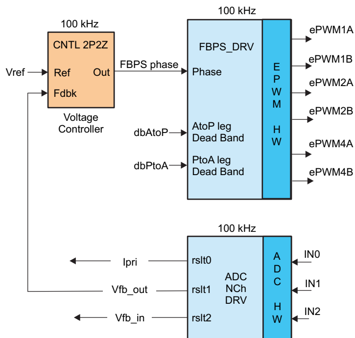
图 13. VMC 方框图
