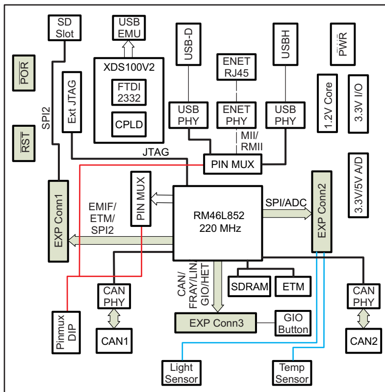
图 1-1. RM46HDK 方框图
