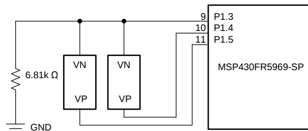
图 2. LMT01-SP to MSP430FR5969-SP Biasing
