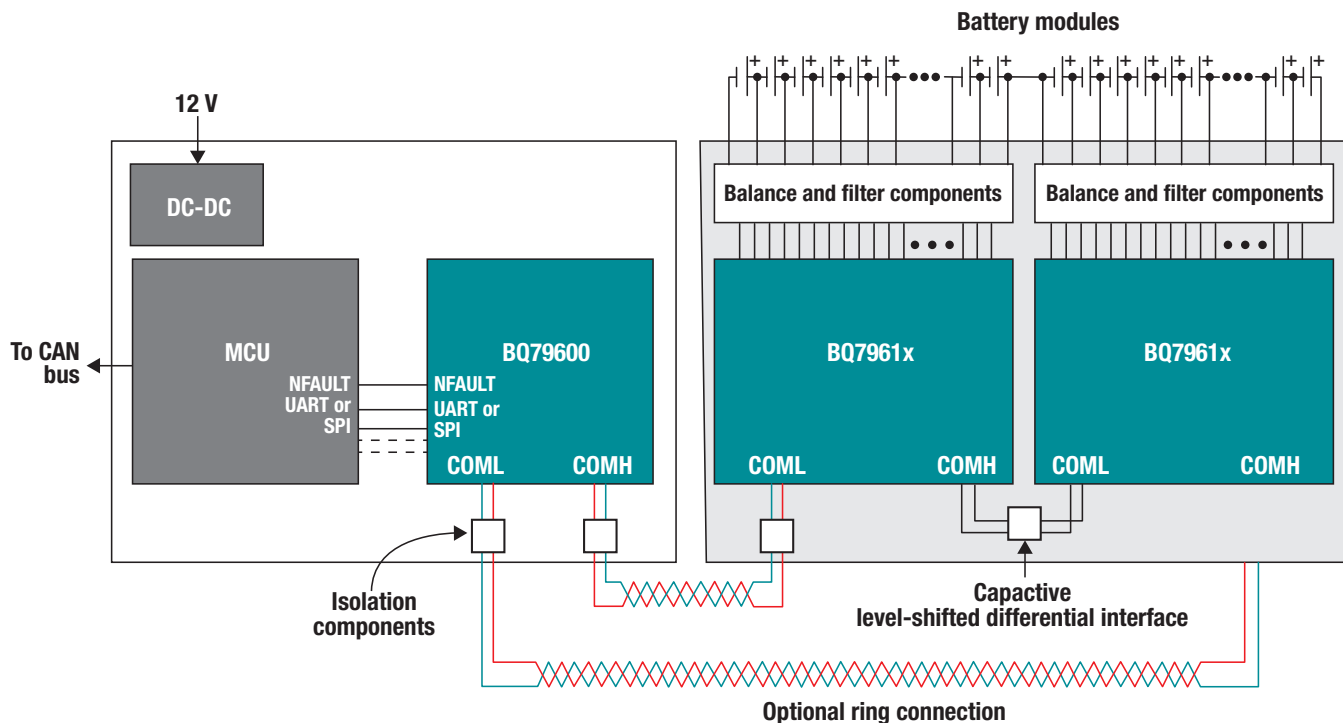
图 3.通过 BQ79616 实现的双向环网配置。
